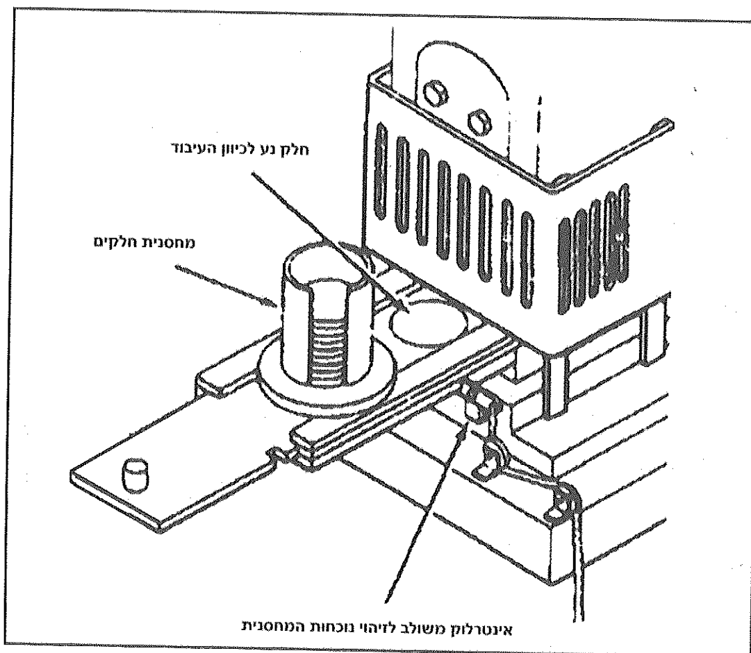
איור 10: המכונה לא תפעל כל עוד המגש מצוי מחוץ למקומו
