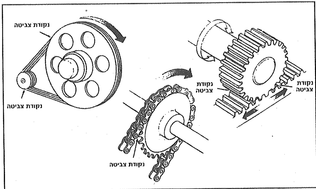
איור 3: חלקים סובבים וחלקים הנעים במשיק להם
