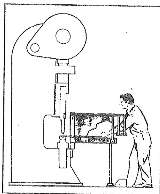
איור 13: מגן מירווח לפני נקודת העיבוד במכונה
