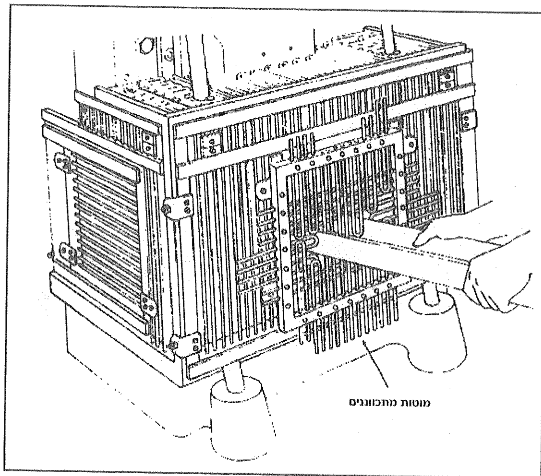
איור 12: מוטות מתכווננים במגן קבוע להגנה על נקודת העיבוד הפעילה
